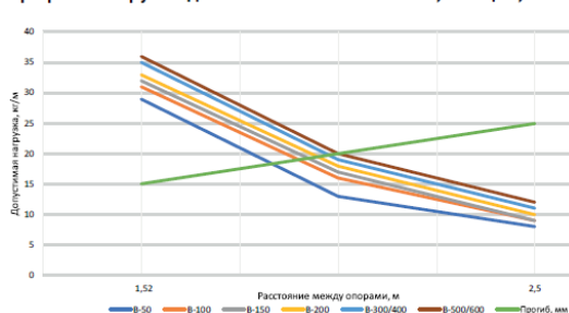
Графики нагрузок для лотков высотой 50 мм, толщ. 3,8 мм
