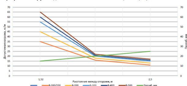
Графики нагрузок для лотков высотой 30 мм, толщ. 4,8 мм
